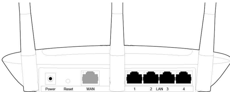
图 3-2 TL-WR885N 端口示意图
