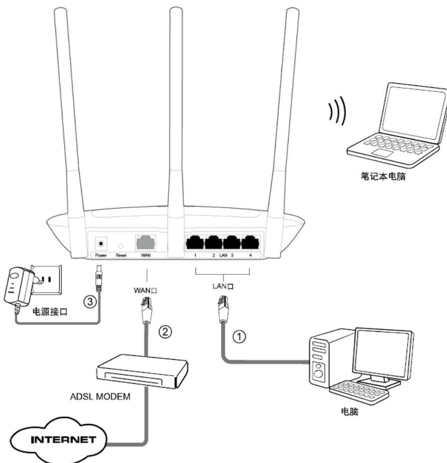
图 4-1 TL-WR885N 硬件安装示意图
