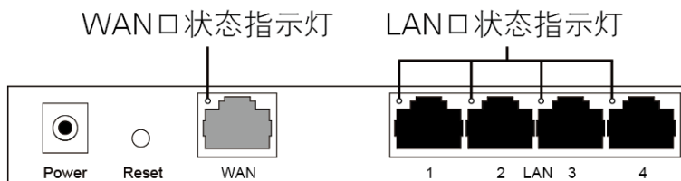
图 3-1 TL-WR885N 指示灯示意图
